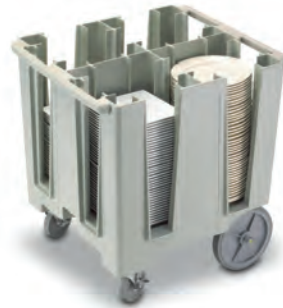
Carro portaplatos no ajustable DCS950 gris. Cambro Ref. Tamaño Capacidad 0101206 69 x 78 x 81 cm Para 225 a 300 platos *para platos de 21,3 a 24,1 cm ø.
