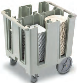
Carro portaplatos no ajustable DCS1125 granito. Cambro Ref. Tamaño Capacidad 0902645 69 x 78 x 81 cm. Para 180 a 240 platos *para platos redondos de 24,4 a 28,6 cm ø y cuadrados de 21,3 a 24,1 cm.
